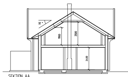
SEKTION AA
