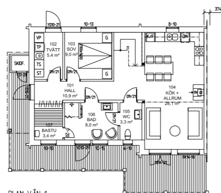
PLAN VÅN 1
