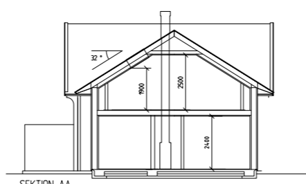
SEKTION AA
